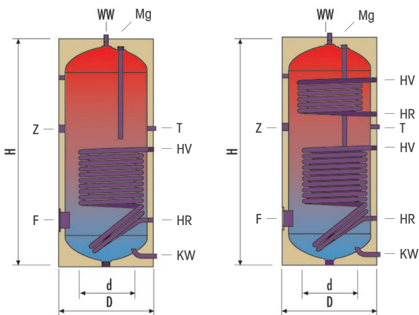
Provedení se solárním zařízením se 2 výměníky tepla s hladkými trubkami.
